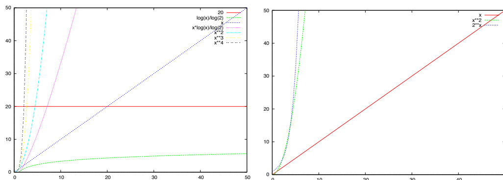
FIGURE 1.2 – Représentation graphique de quelques fonctions usuelles
