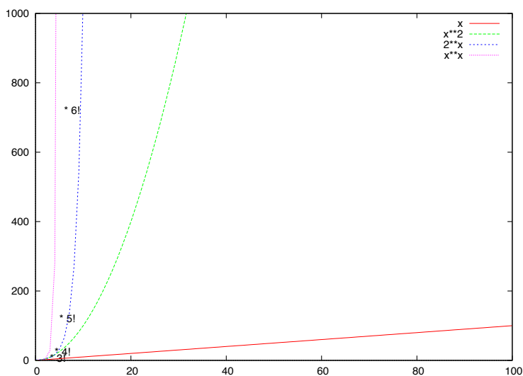
FIGURE 1.3 – Représentation des fonctions de grande complexité (repère non normé)
